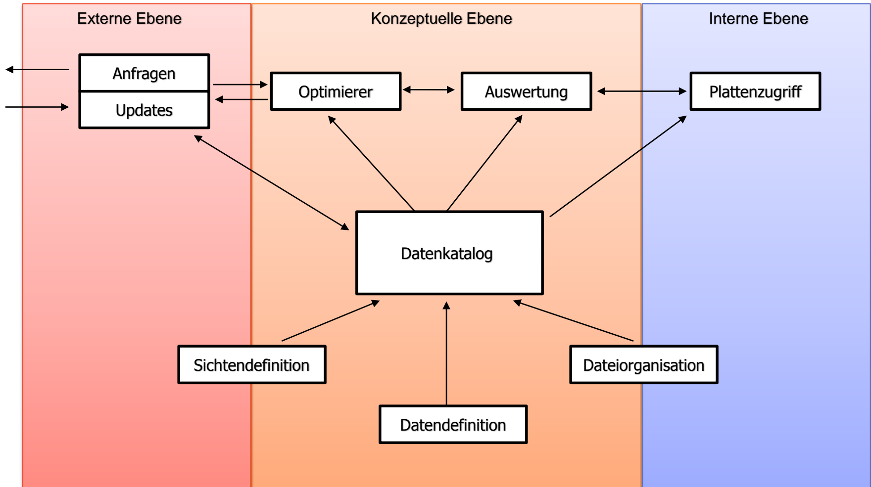
ANSI-SPARC 3-Ebenen-System-Architektur
