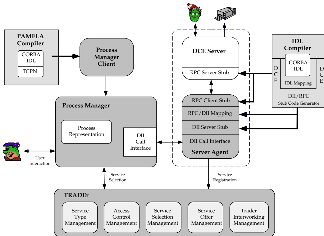
Abbildung 3: TRADE-Gesamtarchitektur
