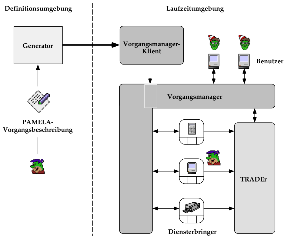
Abbildung 1: TRADE-Gesamtarchitektur
